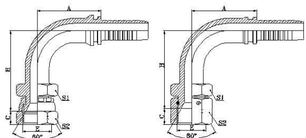
90° 日本公制内螺纹 60° 内锥面 90° JIS METRIC FEMALE 60° CONE SEAT
