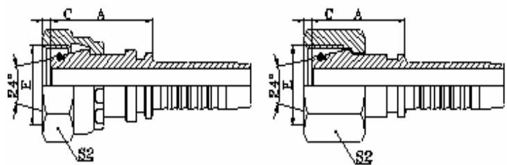
公制内螺纹 24°锥带 O 形圈轻系列 ISO 2151-2-DIN 3865 METRIC FEMALE 24° CONE O-RING L.T.
